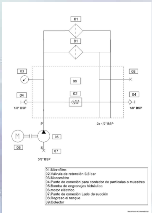
Esquema Hidráulico OLFS
